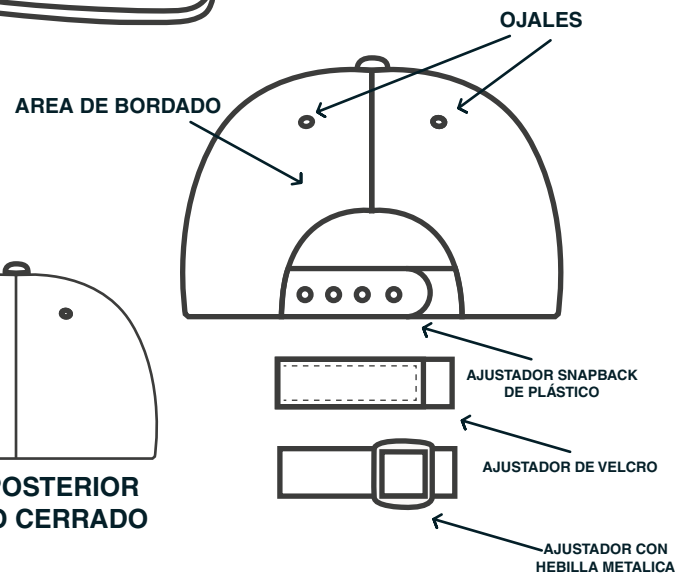
VISTA POSTERIOR
